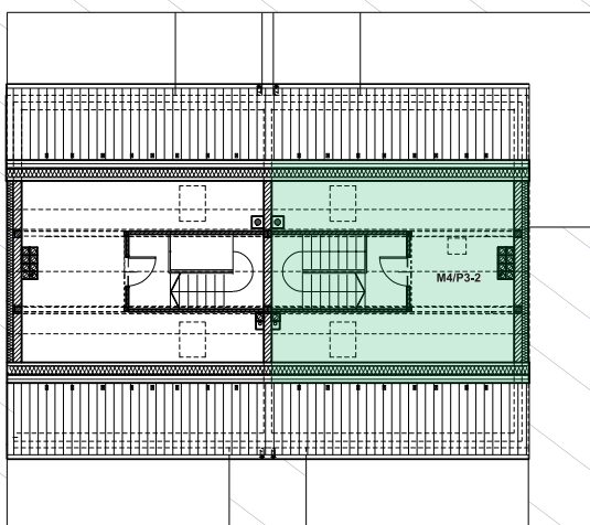
RZUT PODDASZA
