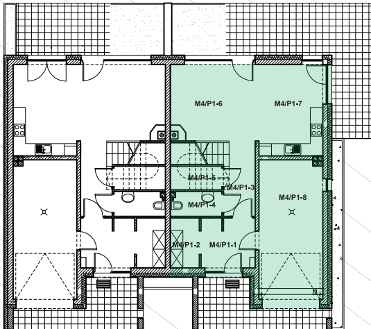
RZUT PARTERU
