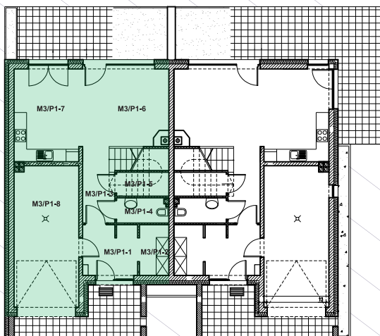
RZUT PARTERU
