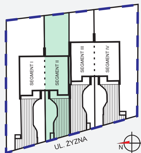
ZAGOSPODAROWANIE TERENU
